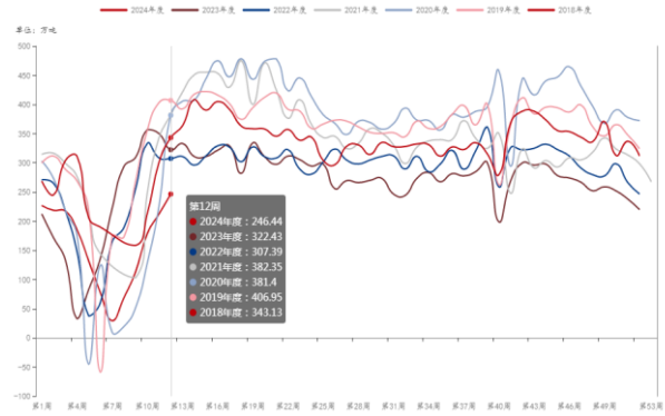
图 2. 螺纹钢表需小幅回升（万吨）
