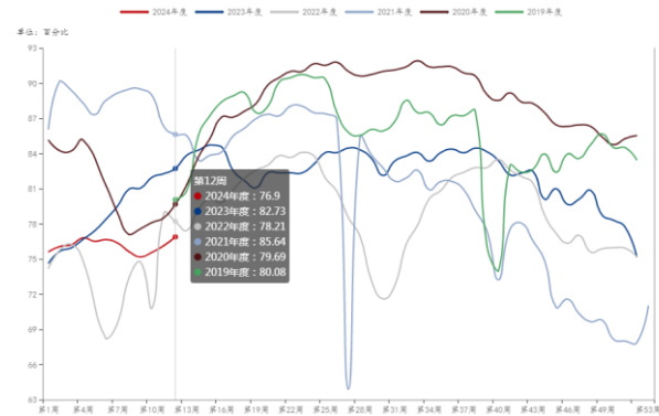
图 4. 高炉开工率处于近年低位（%）
